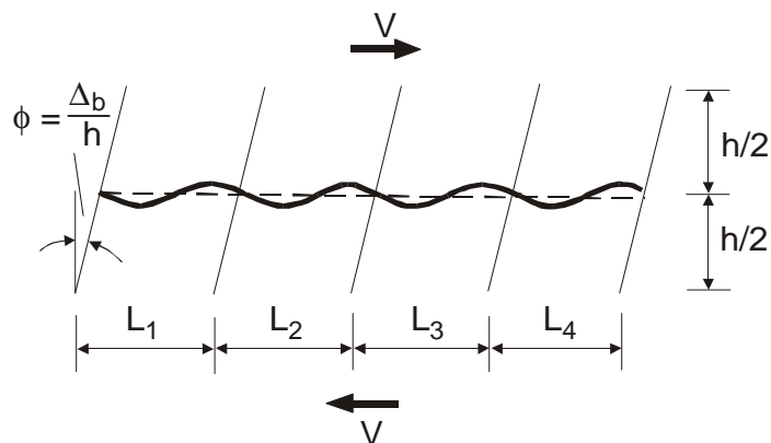
Rys. 1. Przechył ramy od zginania rygli
